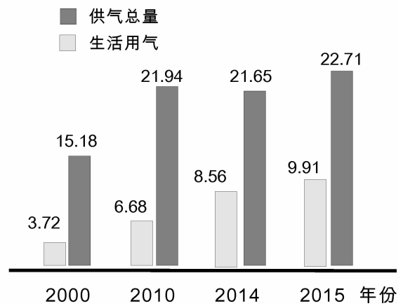
城市供天然气量 (亿立方米)
